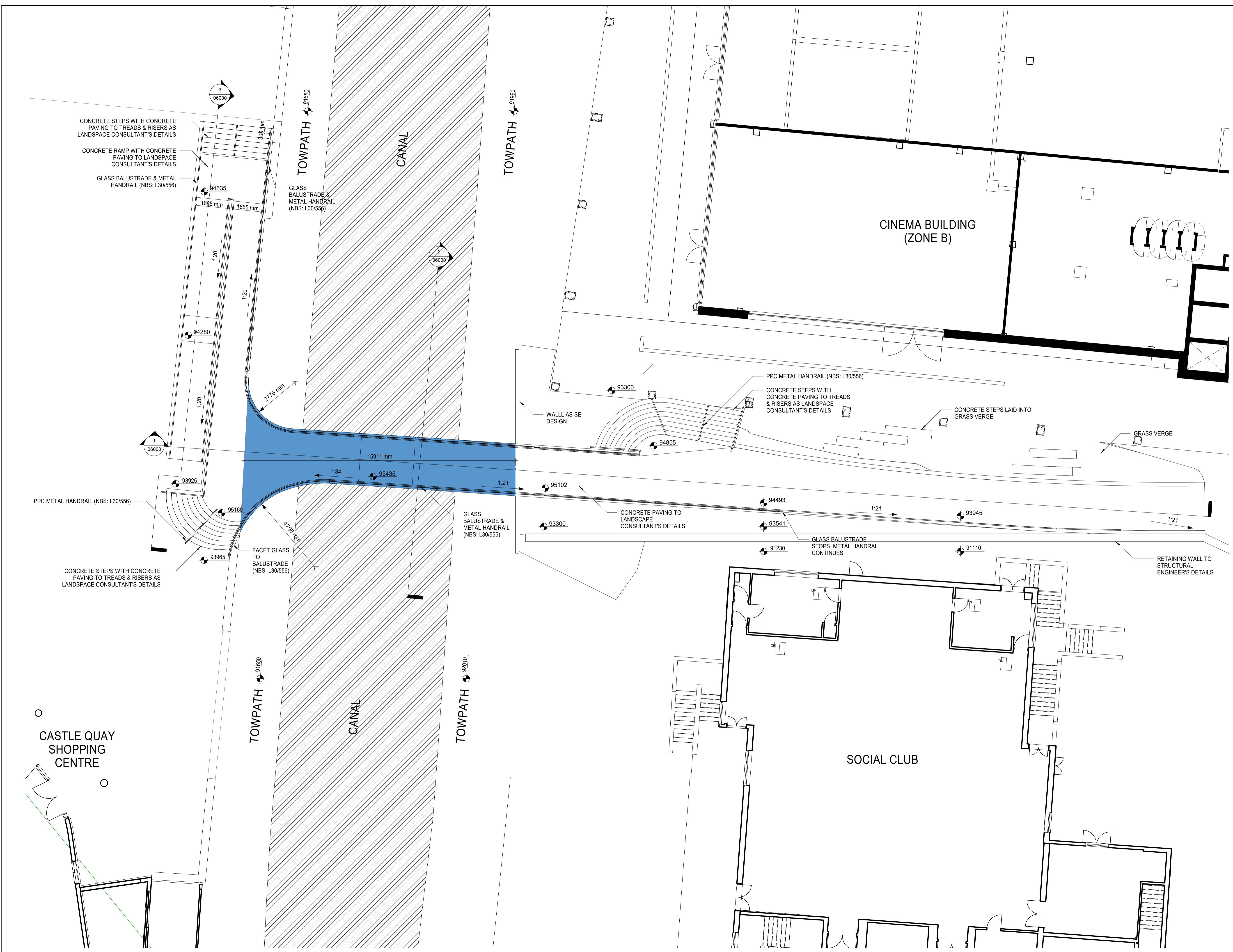
1 FOOTBRIDGE PLAN 1 : 100
